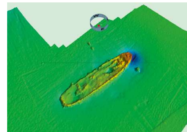
Рис. 6а. Гидроакустическое изображение останков трехмачтового парусника на дне, полученное с помощью многолучевого эхолота. Из архива ЦПИ РГО
