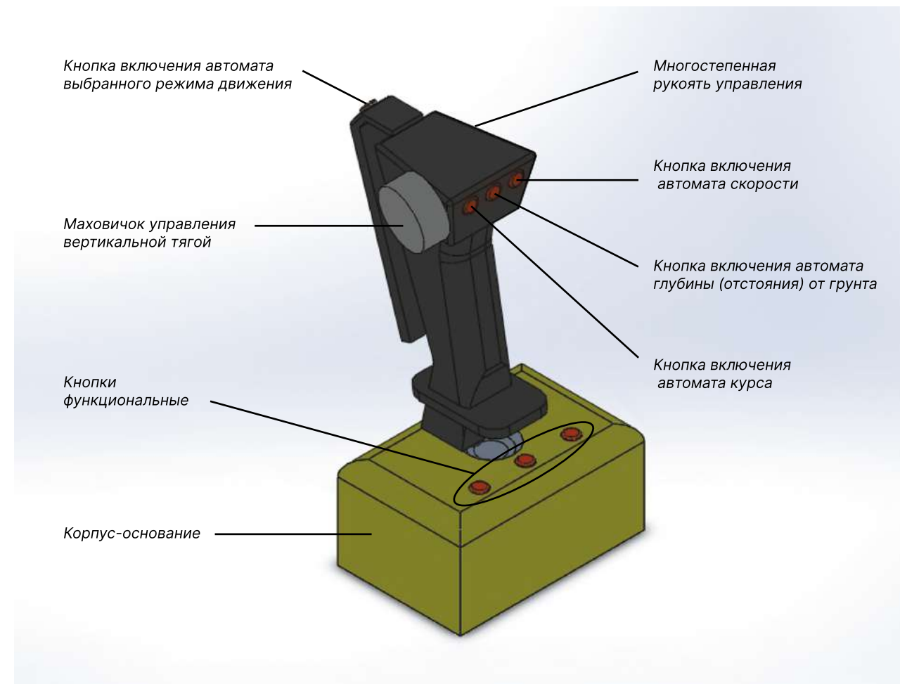
Рис. 3. Вид универсальной рукояти управления для перспективного ОПА (проект). Из архива ЦПИ РГО
