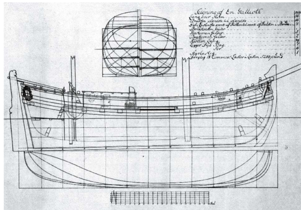
Рис. 2б. Чертеж полуторамачтового голландского гальота. Gronhagen J., Konttinen H. Tietoa syvyyksistä. Hylkytutkimuksen opas. Helsinki: Toredonavalis, 1988. 6, 153 S.
