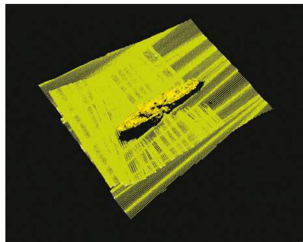
Рис. 3в. Гидроакустическое изображение парохода «Аркона» на дне, полученное с помощью многолучевого эхолота. Из архива ЦПИ РГО
